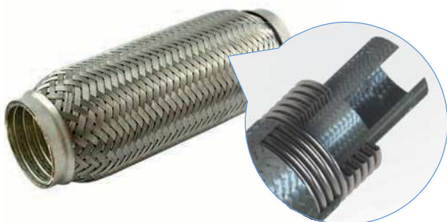
Versione Inner Braid
