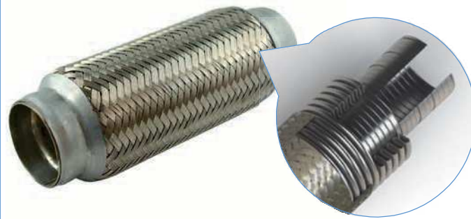
Versione InterLOCK
